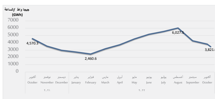
التغير في استخدام الكهرباء، أكتوبر ٢٠٢١ - أكتوبر ٢٠٢٢ Change in Electricity Utilization, Oct. 2021 - Oct. 2022
